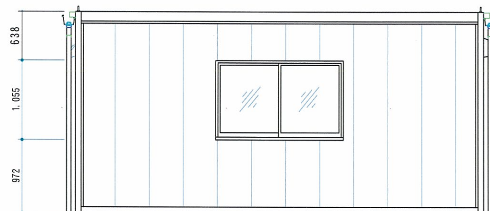
Y 2 立面図 S=1/50
