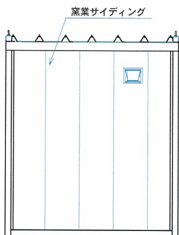
X 1 立面図 S=1/50
