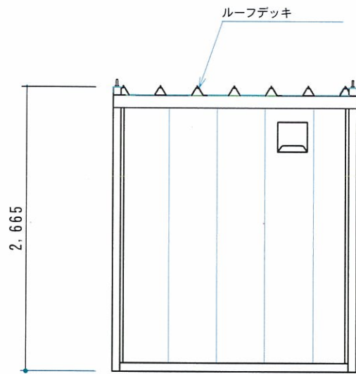
X 1 立面図 S=1/50
