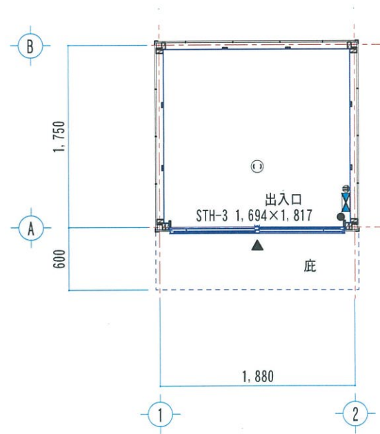
平面図 1:50
