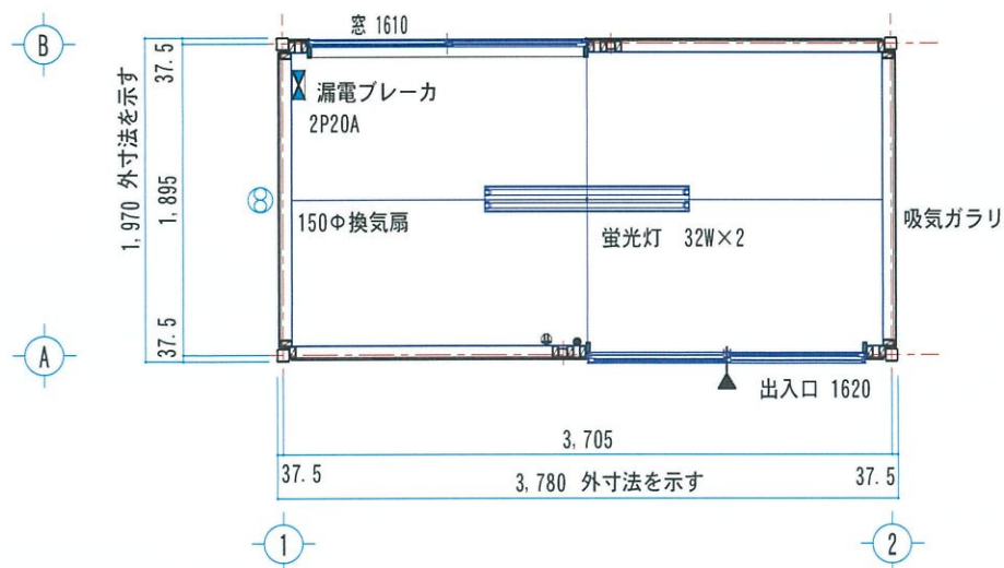
平面図 1:50
