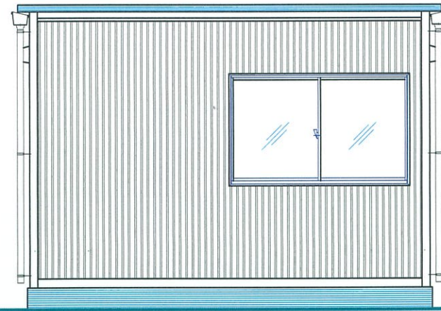
B通り立面図 1:50
