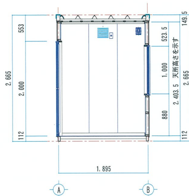
断面図 1:50
